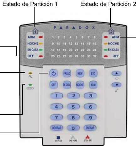
Figura 3: MG32LRF (Módulo Teclado LED Inalámbrico de 32 Zonas)
